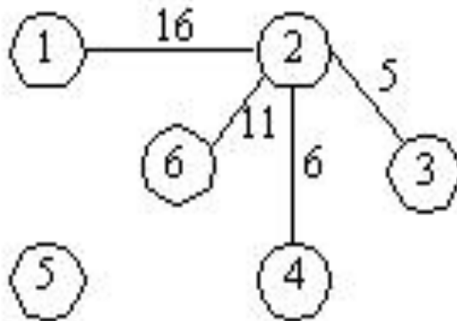
(f) 加入边(1, 2)
