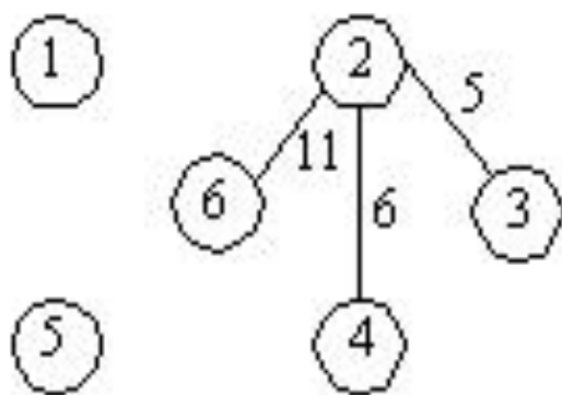
(e) 加入边(2, 6)
