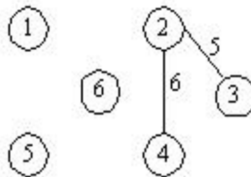
(d) 加入边(2, 4)
